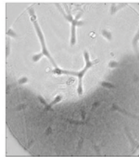
Dissolution du CO 2 dans l'eau à p = 2 Mpa visualisée par Shadowgraphie par le dessous, configuration 3D
