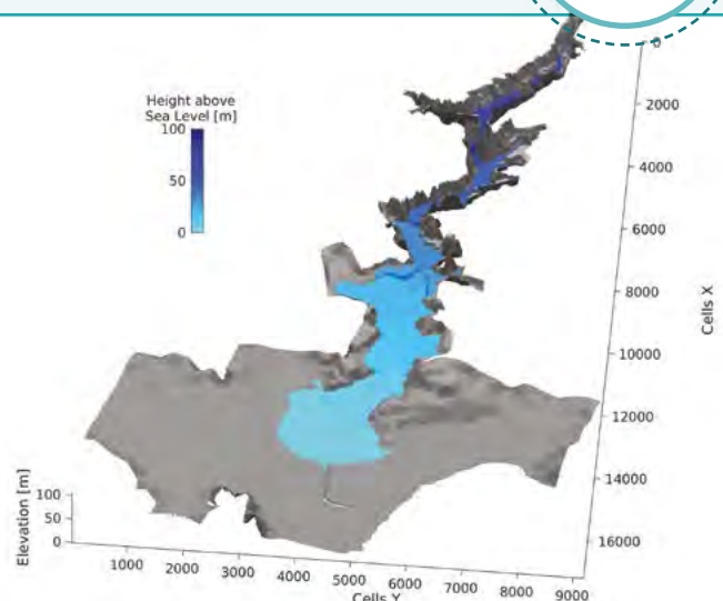
Rupture du barrage de Malpasset calculée grâce au nouveau modèle GPGPU HPC-Waves
